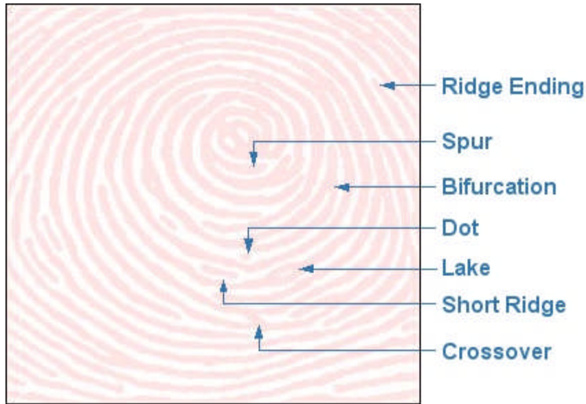
Figure 1 Minutiae Categories
